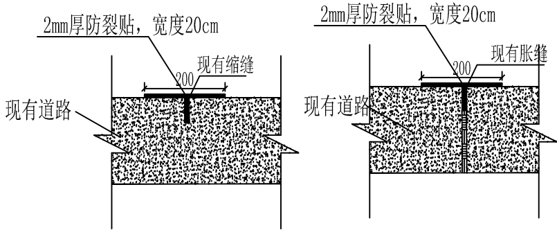
防裂贴示意图
