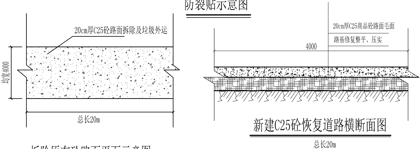
拆除原有砼路面平面示意图 1: 50
