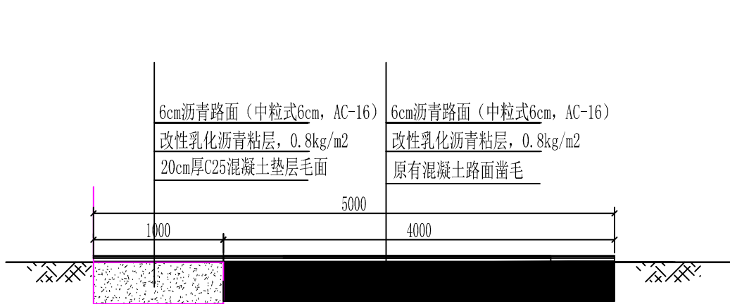
新建5米宽沥青道路横断面图
